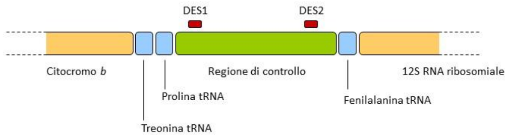
Figura 3. Posizioni di attacco dei primers DES1 e DES2 per l'amplificazione di una porzione parziale della regione di controllo del DNA mitocondriale relativamente ad altri geni contigui (vedi testo per ulteriori dettagli).
